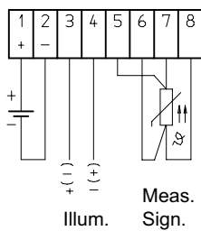
Typ -PxL4, -PTxL4 (4-Leiter)
