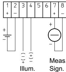
Typ -I1, -I2, -I0, Typ -U1, -U2, -U0
