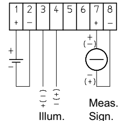
Typ PxL3, Typ PTxL3 (3-Leiter)
